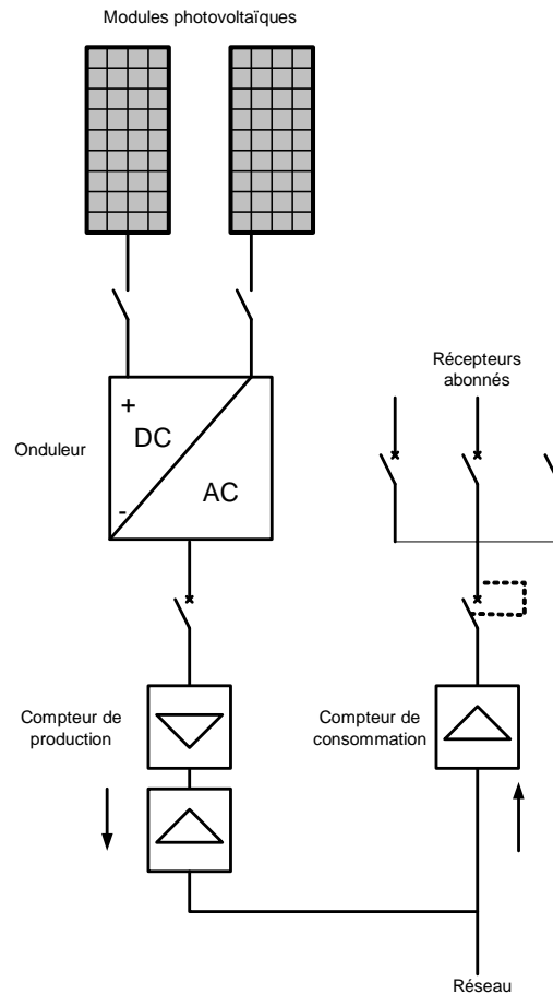
Synoptique du KYOCERA 2940
